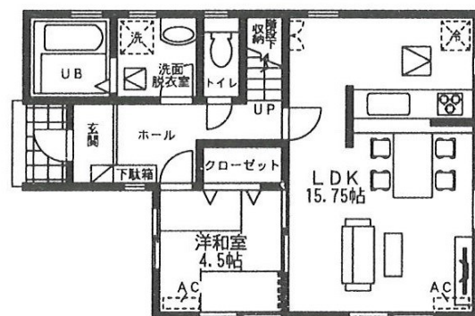
1階平面図: 51.76m 2
